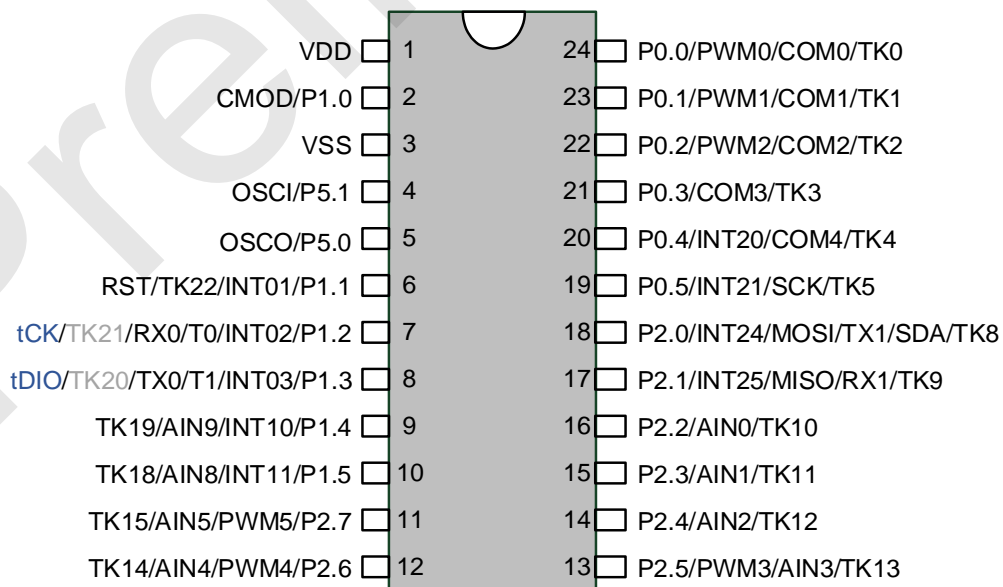
SSOP24 管脚配置图
