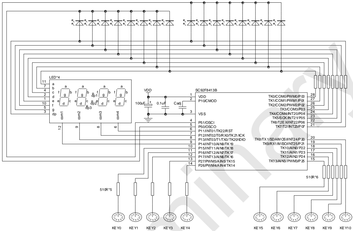
SC92F8413B Touch Key 应用电路图
