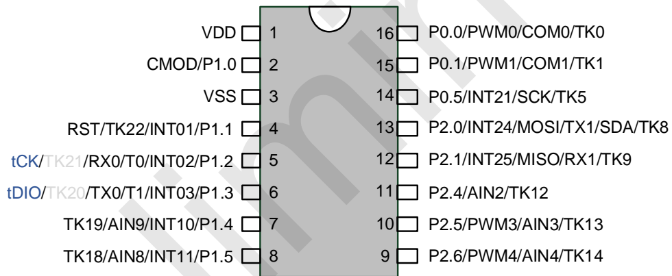
SOP16 管脚配置图
