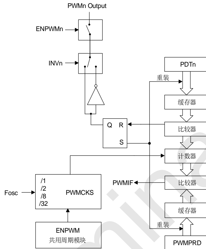
SC92F841XB PWM 独立模式框图
