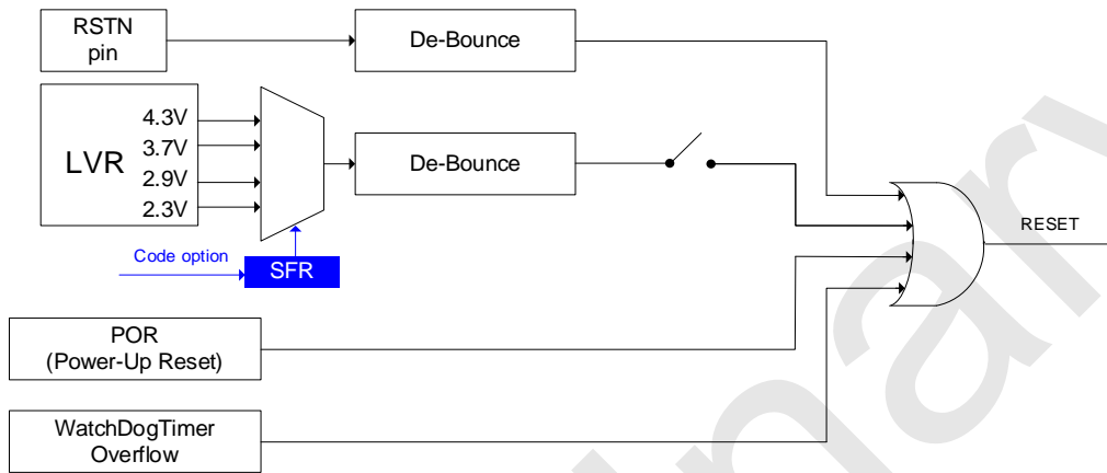
SC92F841XB 复位电路图
