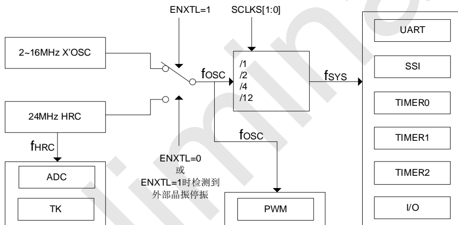
SC92F841XB 内部时钟关系
