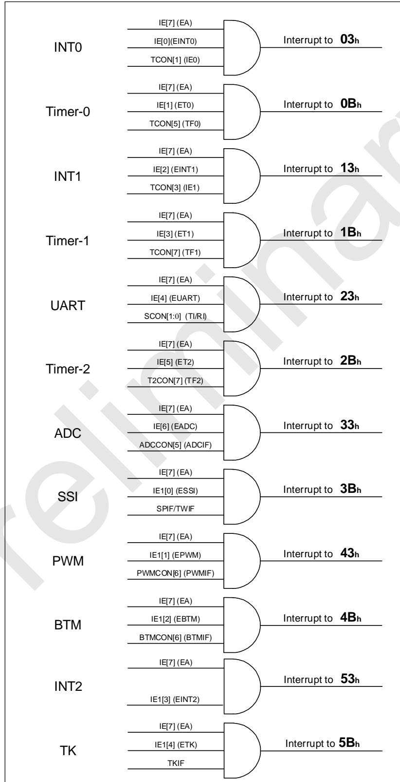
SC92F841XB 中断结构和向量
