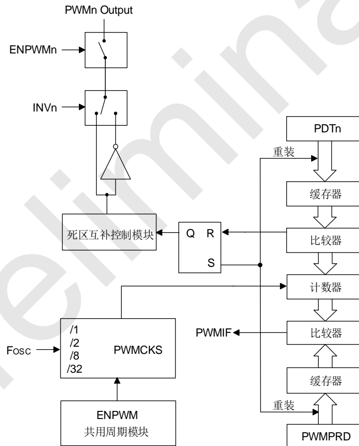
SC92F841XB PWM 结构框图
