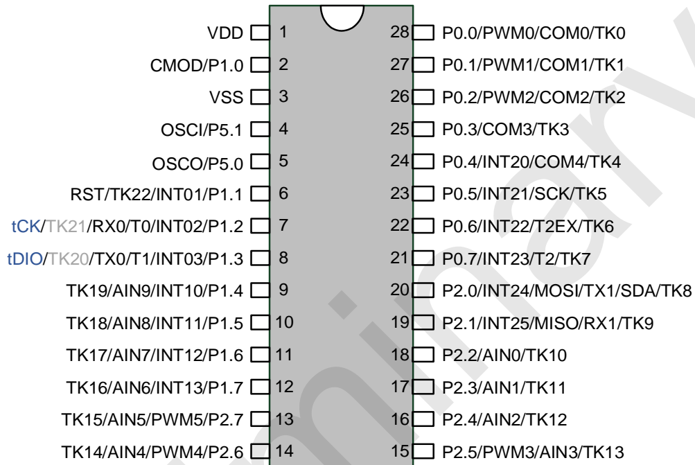
SOP28/TSSOP28 管脚配置图
