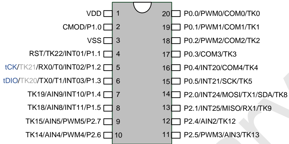
SOP20/TSSOP20 管脚配置图
