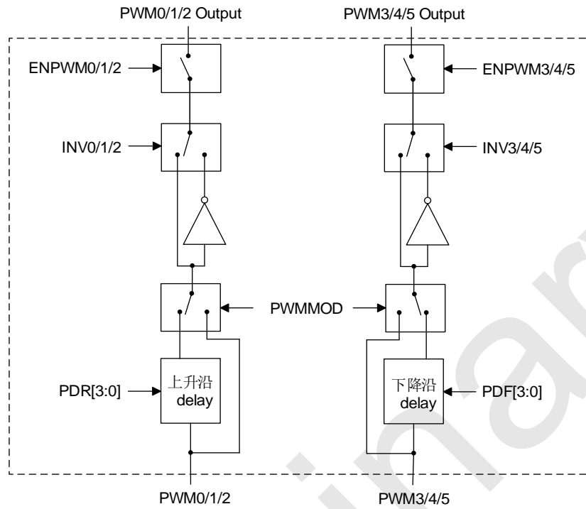
SC92F841XB PWM 互补模式框图
